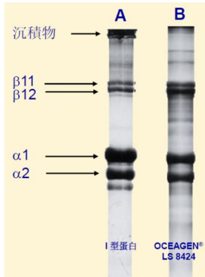
電泳圖
